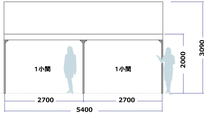
【立面図】
